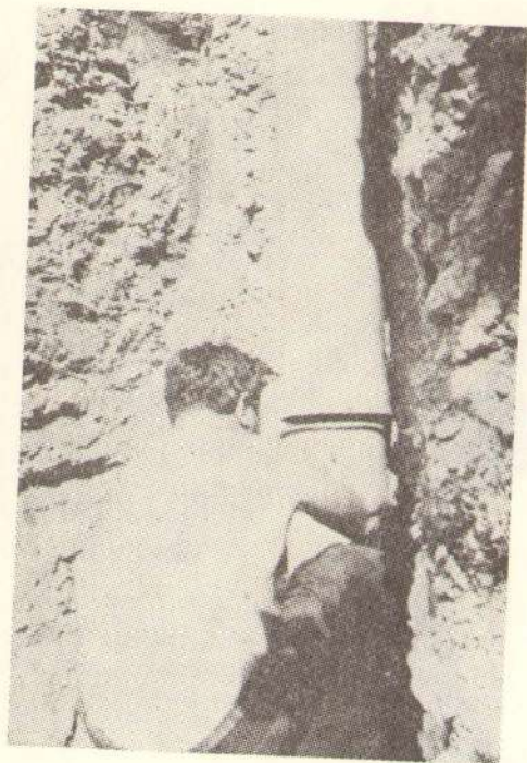
Сл. 11 Спајање RAUDRIL-DK цеви DN 250 помоћу O-бртвила
