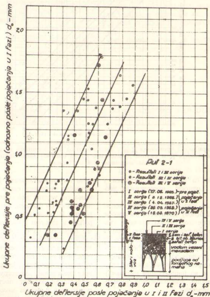
Сл. 7 — Однос укупних дефлексија d_0 измерених на површини коловозног вастора пре и после обављених радова на појачању у I и II фази, на опитној деоници бр. 2
