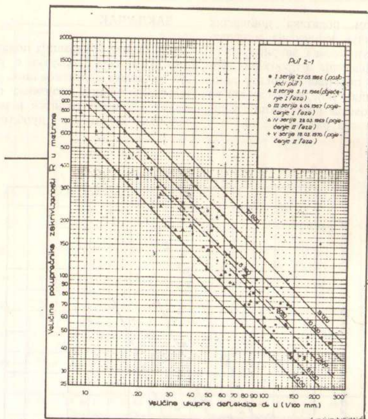
Сл. 8 — Варијације производа R d_0 у зависности од полупречника закривљености линије дефлексија R и укупне дефлексије d_0 на опитној деоници бр. 2, пре и после појачања у I и II фази
