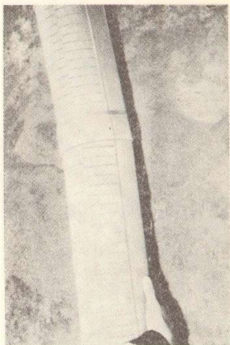
Сл. 2 Припрема KAUDRIL-D цеви преа спајањем — увек у правцу тока воде
